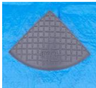
●渡り石(コーナー用)300×300×H100
