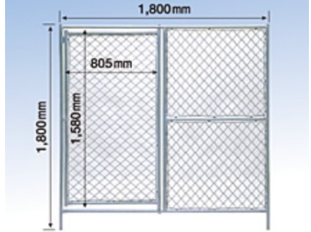
●フェンスバリケード 潜戸付 1800×1800
